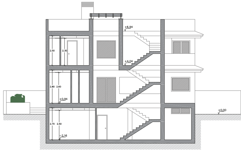
SECCIÓN A-A
